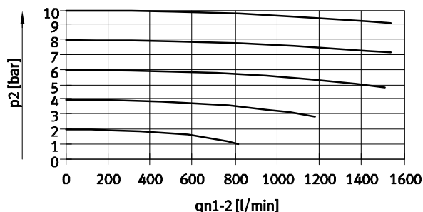
Caudal q_{n1 \rightarrow 2} en función de la presión de salida p_2
