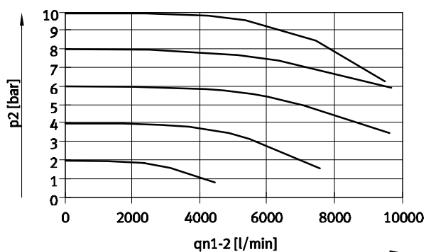
Caudal q_{n1 \rightarrow 2} en función de la presión de salida p_2
