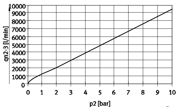
Caudal q_{n2 \rightarrow 3} en función de la presión de salida p_2
