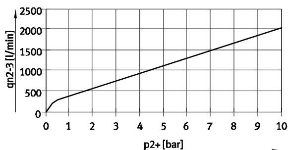
Caudal q_{n2 \rightarrow 3} en función de la presión de salida p_2
