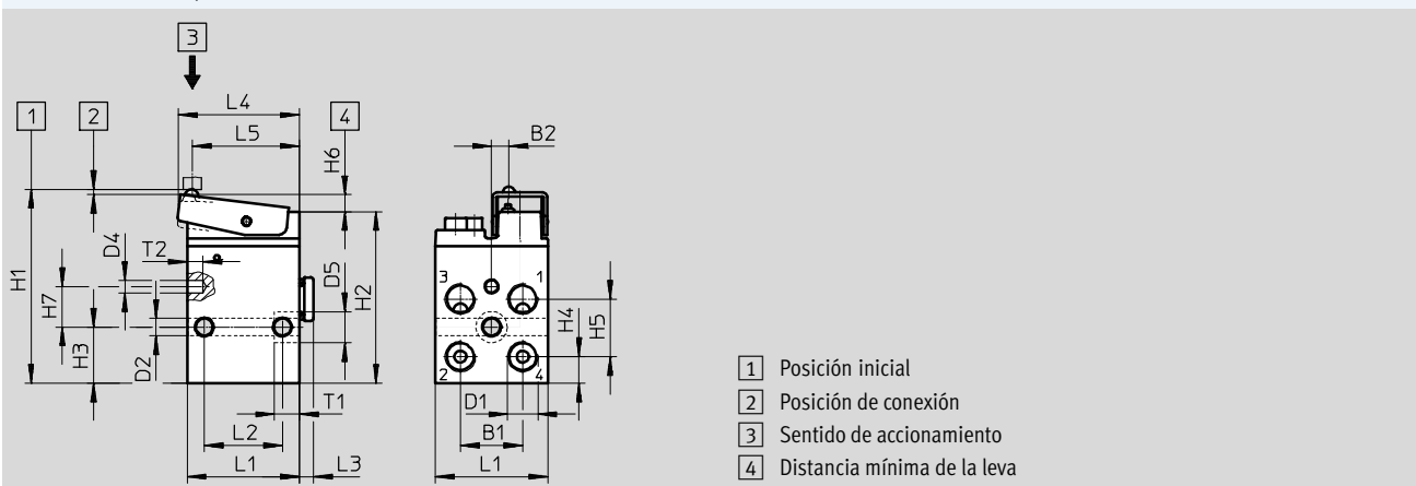
Válvula de leva VS-4-1/8
