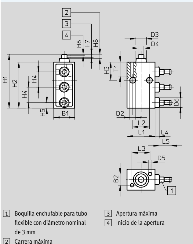
Válvula de leva V/O-3-PK-3
