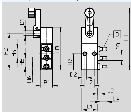
Válvula con palanca basculante RW/O-3-PK-3
