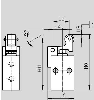
Válvula con rodillo R-3-M5
