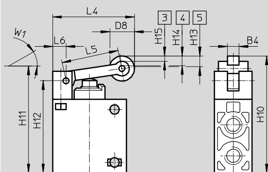
Válvula con rodillo R-3-1/4-B, R0-3-1/4-B
