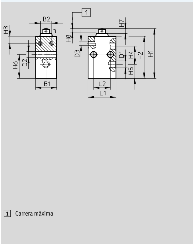
Válvula de leva V-3-M5
