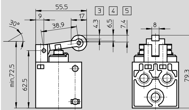
Válvula con rodillo R-5-1/4-B
