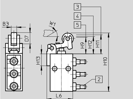
Válvula con rodillo R/O-3-PK-3
