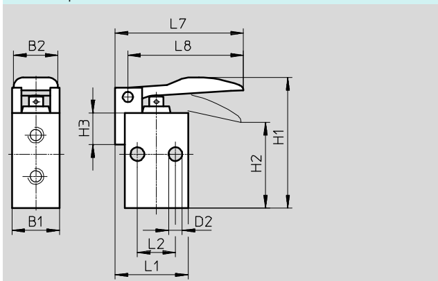
Válvula de palanca TH-3-M5
