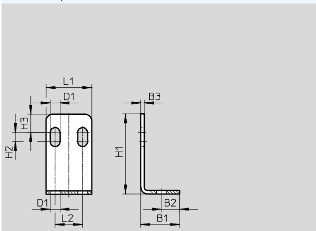
Escuadra de fijación HV-M5
