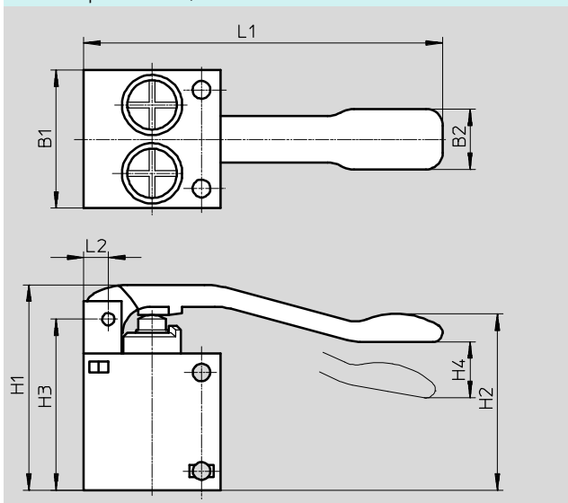
Válvula de palanca TH-5-1/4-B
