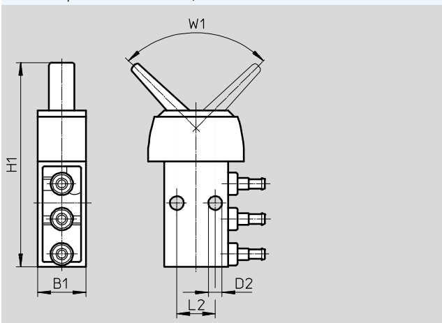
Válvula de palanca basculante KH/O-3-PK-3
