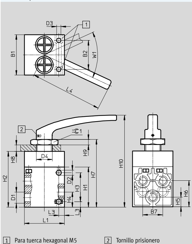
Válvula de palanca manual H-5-1/4-B
