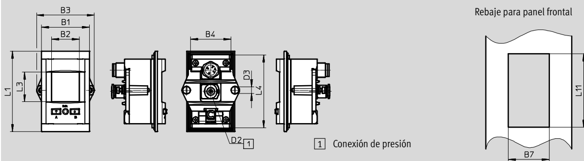
SPAU-...-F-...-MxD
