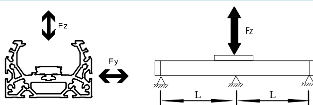
Fuerza Fz
