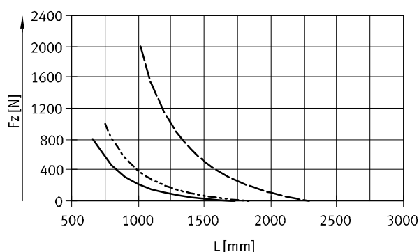
Fuerza Fz
