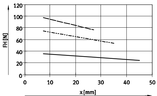
HGPS-35-A
