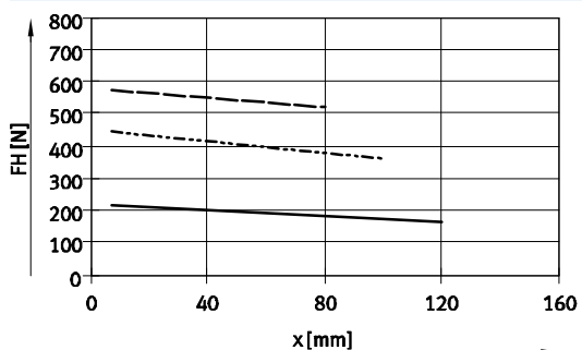
HGPS-80-A
