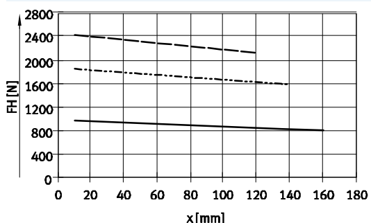
HGPS-80-A
