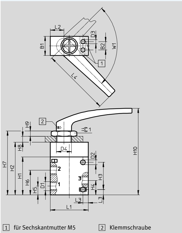
Handhebelventil H-3-¼-B
