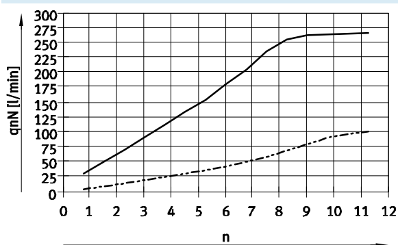
Normalnennendurchfluss q_{nN} bei 6 → 5 bar in Abhängigkeit der Spindelumdrehungen n
