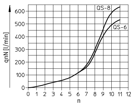
Normalnennndurchfluss qnN bei 6 bar → 5 bar in Abhängigkeit der Spindelumdrehungen n
