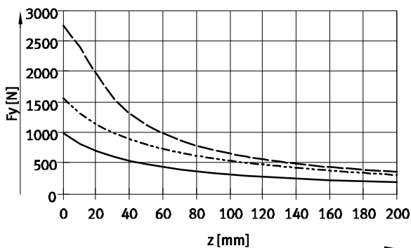
Max. Radialkraft F_y , statisch
