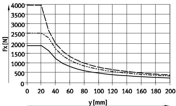
Max. Axialkraft F_x , statisch, drückend und ziehend
