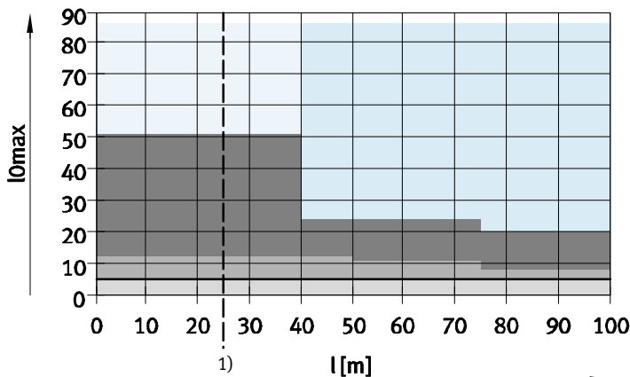
Empfohlener Leitungsquerschnitt in Abhängigkeit der Leitungslänge l und max. Motorstrom I 0
