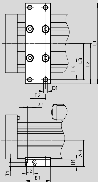
Baugröße 70, 80
