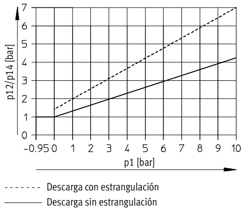
VL/O-3-3/4: posición inicial cerrada
