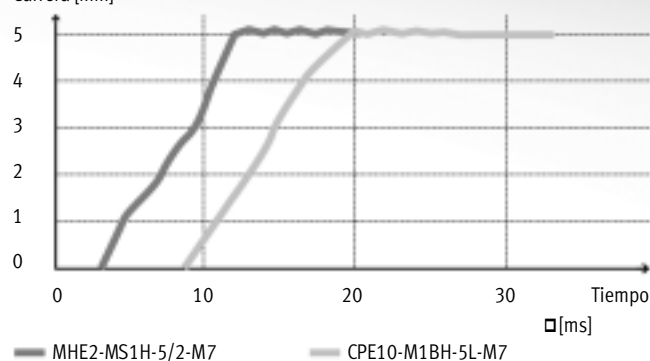
Cilindros de carrera corta ADN-32-5 - 30 % más veloz con válvula de respuesta rápida Carrera [mm]
