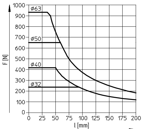
DFM-32 ... 63-GF Carrera 50 mm
