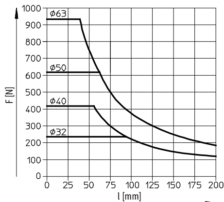
DFM-32 ... 63-GF Carrera 80 ...100 mm
