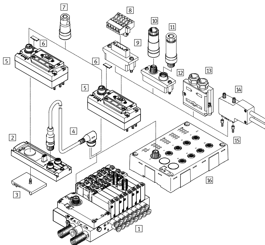
Esquema: CTEU con terminal de válvulas VTUG
