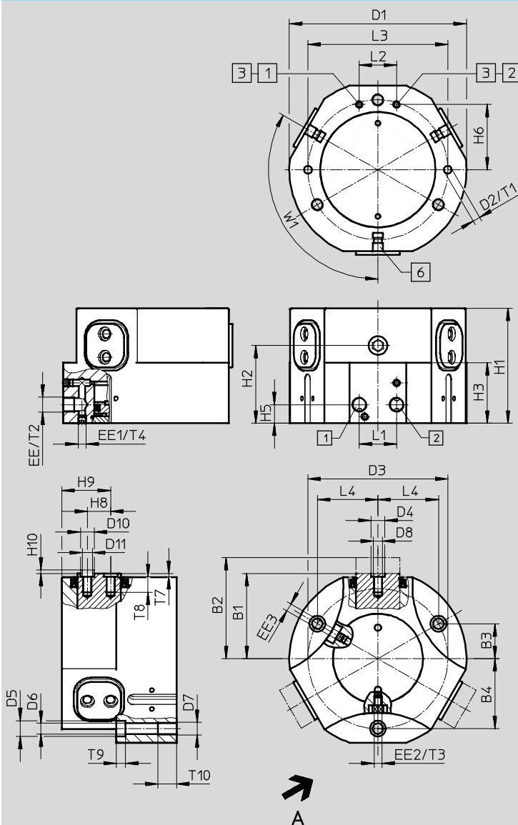
Ansicht A
