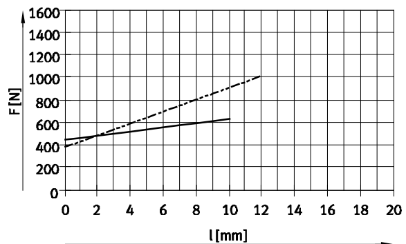
Baugröße 63 ... 80
