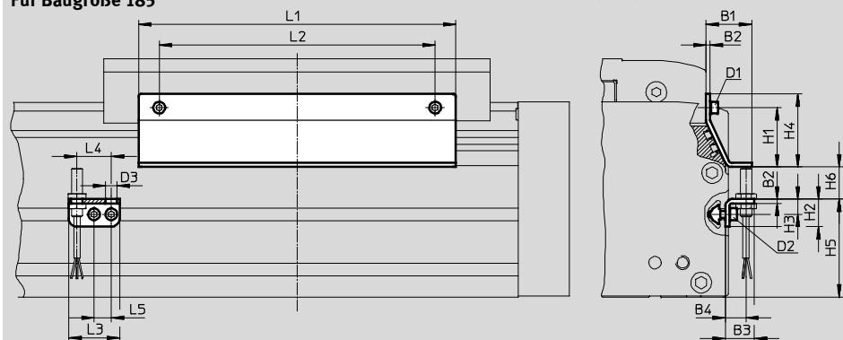
Für Baugröße 185
