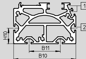
Baugröße 80
