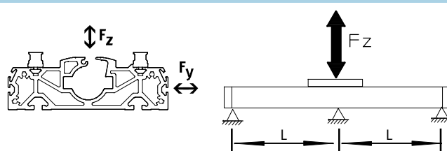
Kraft F_z
