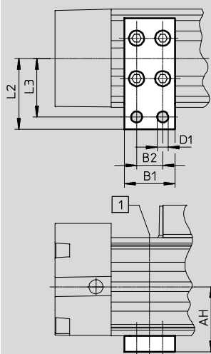
Ø 32 ... 80
