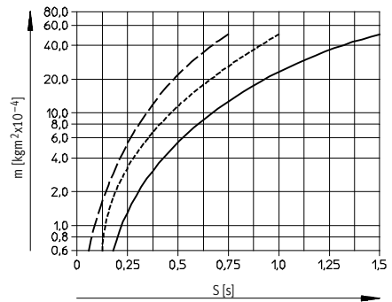
DSR/DSRL-40
