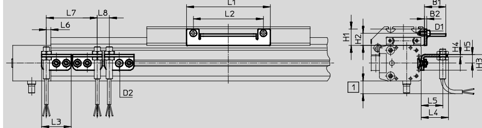
DGE-25-...-ZR-KF-...
