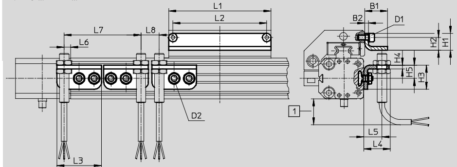
DGE-18-...-ZR-KF-...
