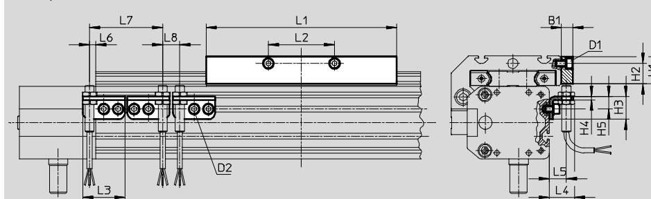
DGE-40/-63-...-ZR-KF-...
