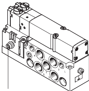
Anschlusstecker M8 x 1, Stift, 4-polig nach EN 60 947-5-2
