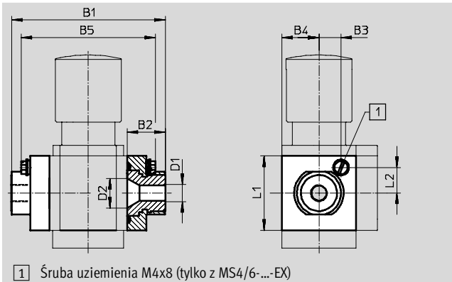
1 Śruba uziemia M4x8 (tylko z MS4/6-...-EX)
