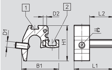
SMBZ-8-125/320
