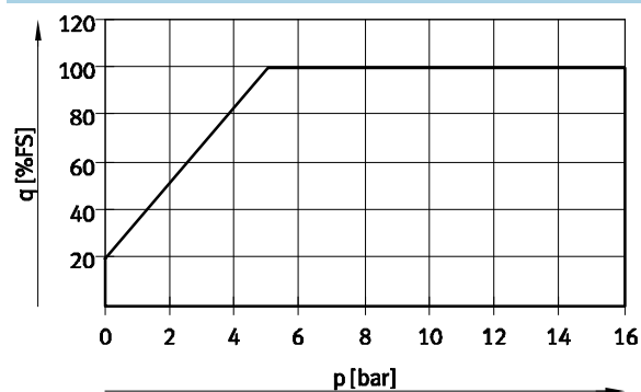
Margen de medición del caudal 1) qn en función de la presión de funcionamiento p1
