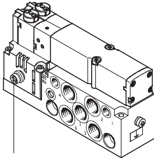
Anschlusstecker M8 x 1, Stift, 4-polig nach EN 60 947-5-2
