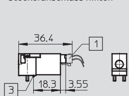
Steckeranschluss hinten
