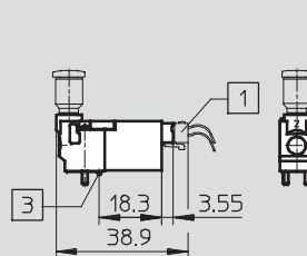
Steckeranschluss hinten
