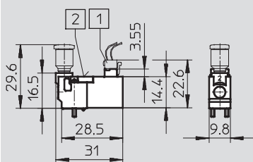
Steckeranschluss oben
