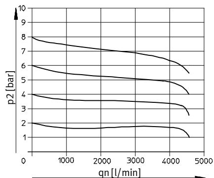
LFR/LFRS- \frac{1}{2} -D-MIDI
