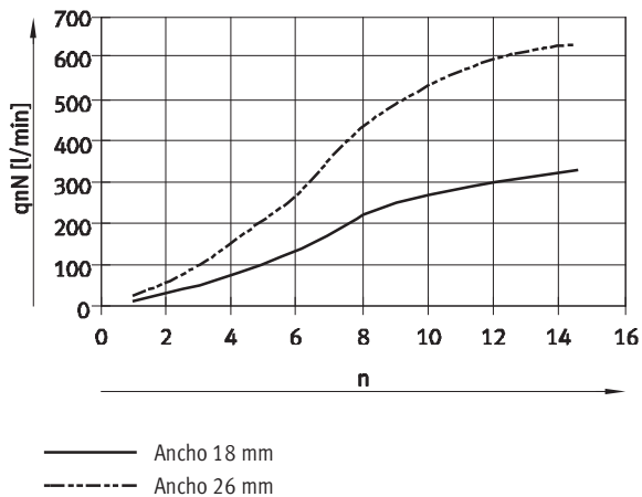
Caudal q_N en función de la estrangulación
