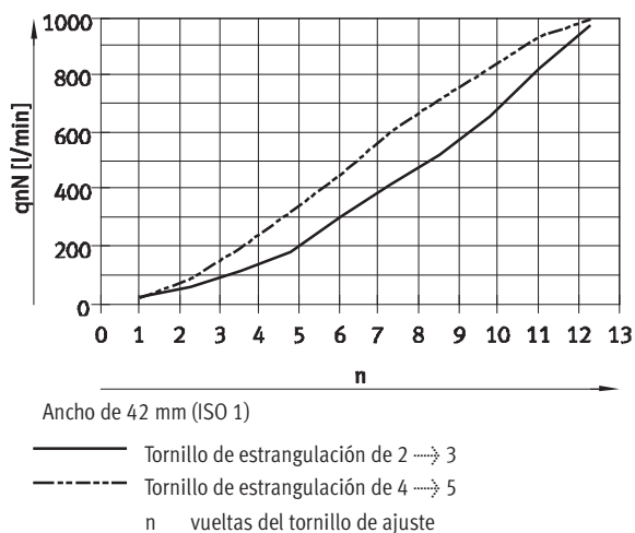
Caudal q_N en función de la estrangulación
