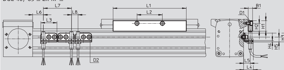
DGE-40/-63-...-ZR-RF-...
