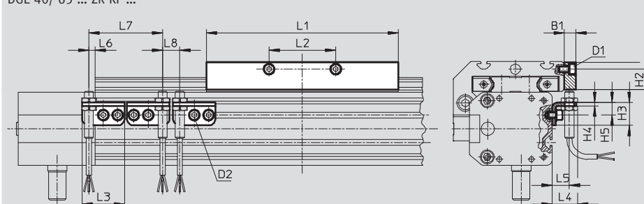
DGE-40/-63-...-ZR-KF-...
