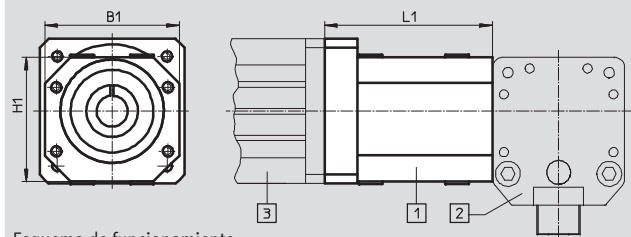
EAMM-A-F-...
