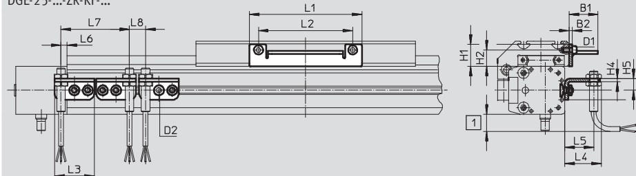
DGE-25-...-ZR-KF-...
