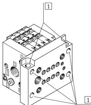
1 Montagebohrungen
