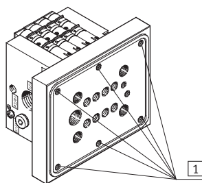
1 Montagebohrungen
