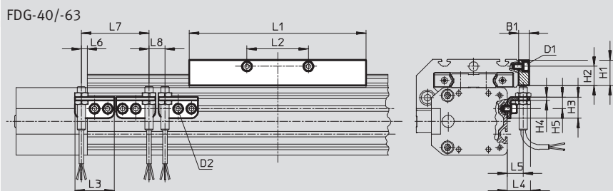
FDG-40/-63
