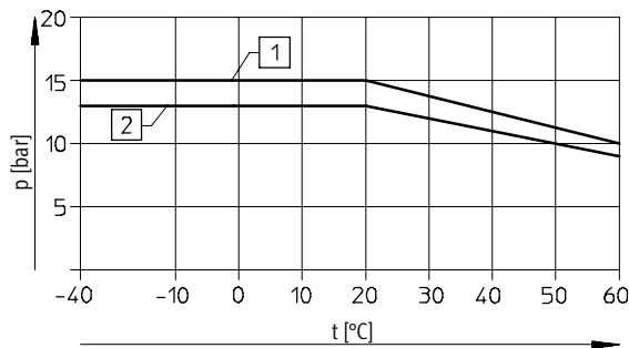
Pression de fonctionnement p en fonction de la température t
