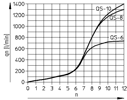
Débit normal qn à 6 bar → 0 bar selon le nombre de tours de vissage n Filetage G3/8
