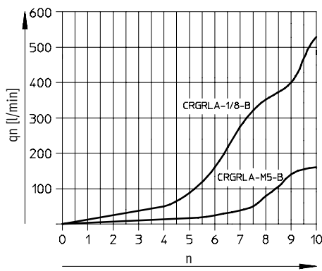
Débit normal q_n à 6 bar → 0 bar selon le nombre de tours de vissage n Filetage M5, G \frac{1}{8}
