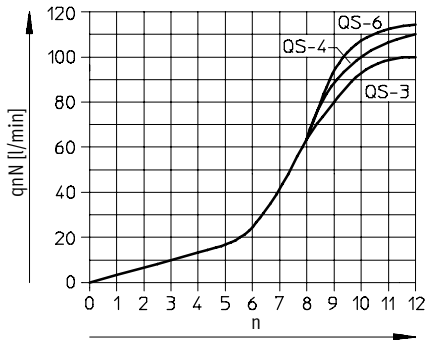
Débit nominal normal qnN [l/min] à 6 bar → 5 bar selon le nombre de tours de vissage n Filetage M5
