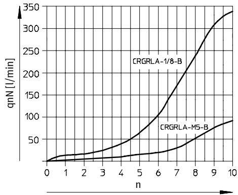
Débit nominal normal q_{nN} à 6 bar → 5 bar selon le nombre de tours de vissage n Filetage M5, G \frac{1}{8}
