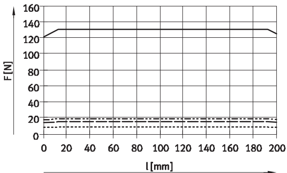
DFME-32-200
