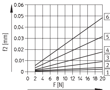
Diámetro del émbolo 10 mm
