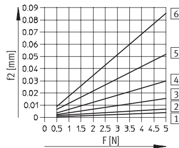
Diámetro del émbolo 6 mm
