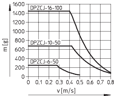
Gleitführung GF
