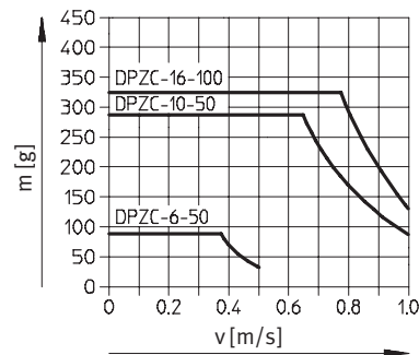
Kugelumlaufführung KF
