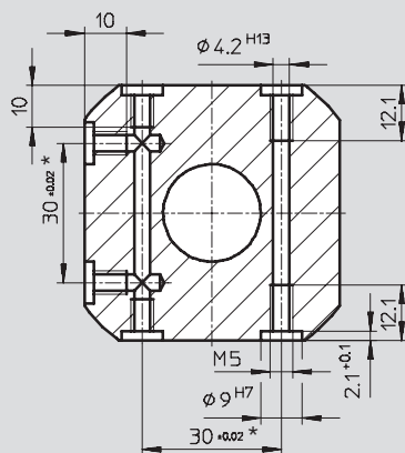
Baugröße 16
