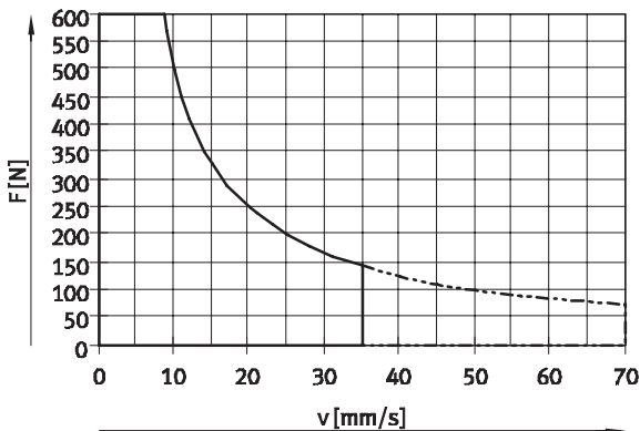
DNCE-40-1...299-LS-...
