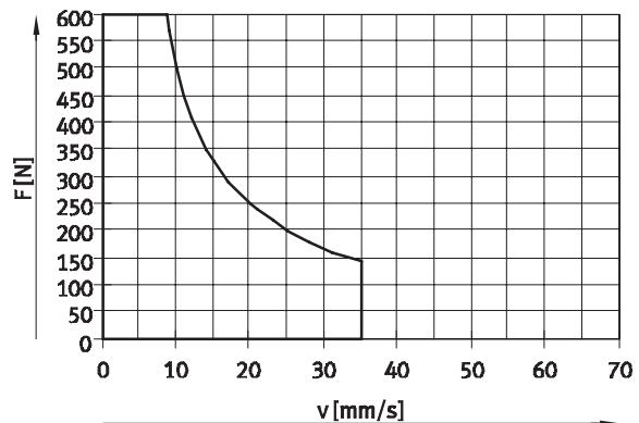
DNCE-40-300...600-LS-...
