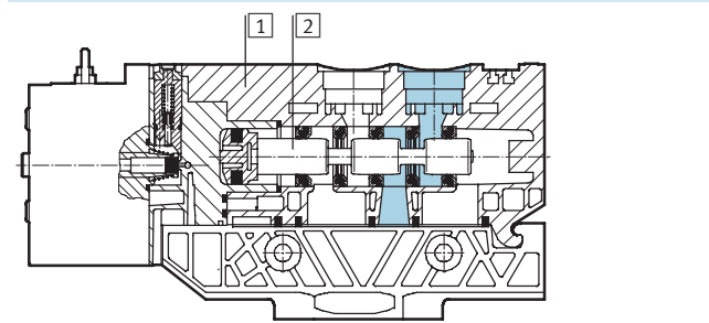
Funktionsschnitt – monostabiles Ventil
