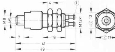
1 Stecknippel für Kunststoffschlauch NW 3 Anschluß P schwarz, Anschluß A gelb
