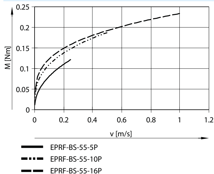
摩擦扭矩 M 与进给速度 v 的关系，用于规格 55
