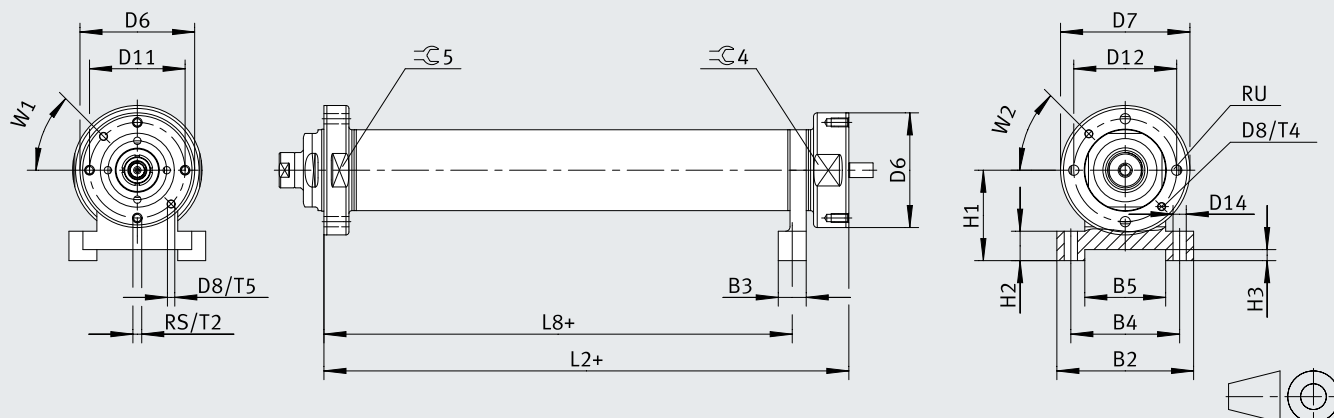
尺寸 - EPRF-...-M6 (带通孔的法兰和脚架安装)
