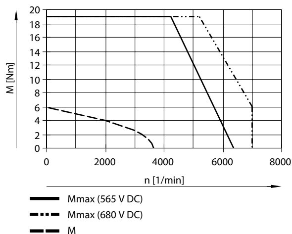
扭矩 M 与转速 n 的关系，用于 EMMH-AS-108-MA-HS-B
