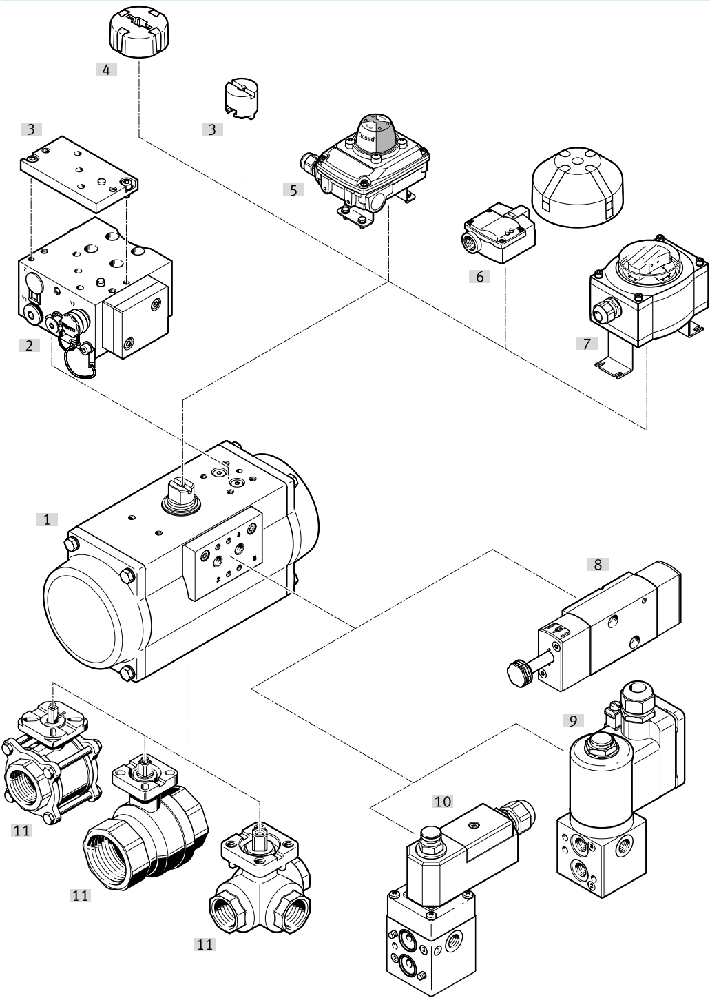
外围元件一览 DFPD-C
