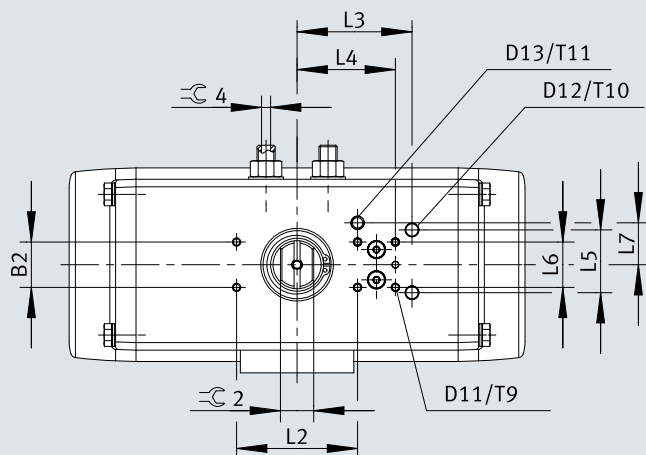
尺寸 - DFPD-C 单作用, 尺寸 20 ...480, 变型 VDE2
