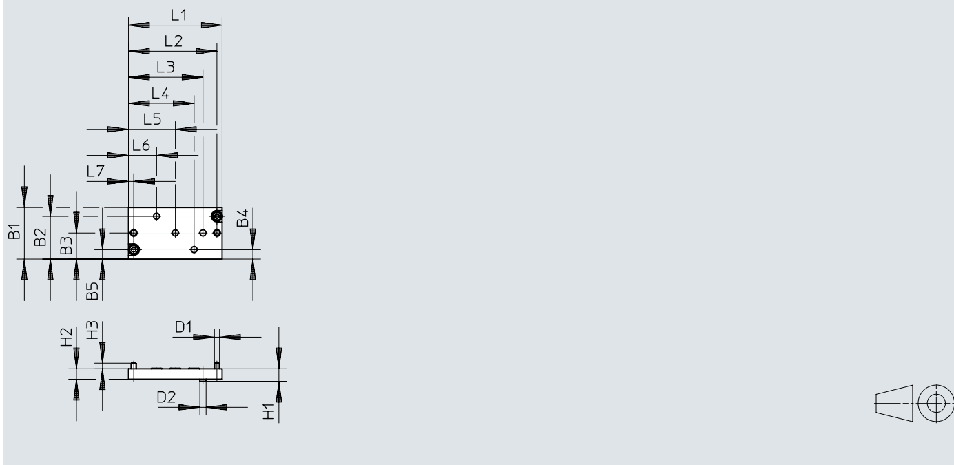
尺寸 – 转接组件 DADG-AK-F9-1
