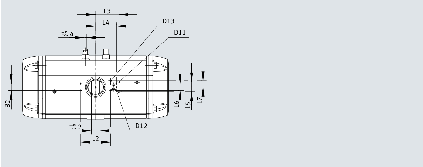
尺寸 – 单作用 DFPD-C, 规格 700 - 2300
