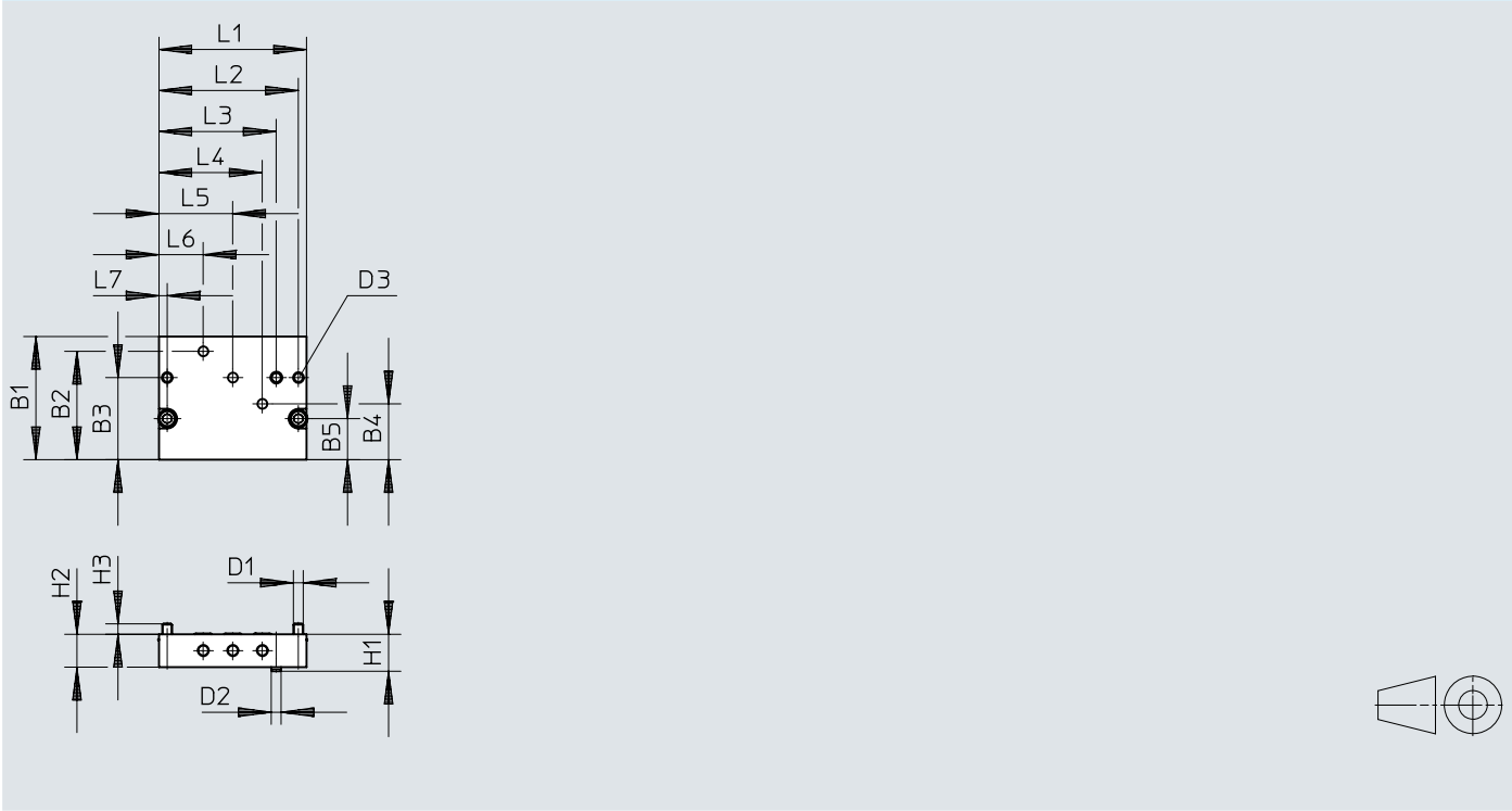
尺寸 – 转接组件 DADG-AK-F9-2
