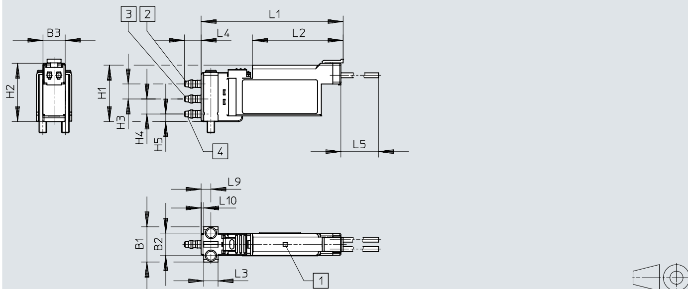
Dimensões – Válvula individual com espigões, conector H5
