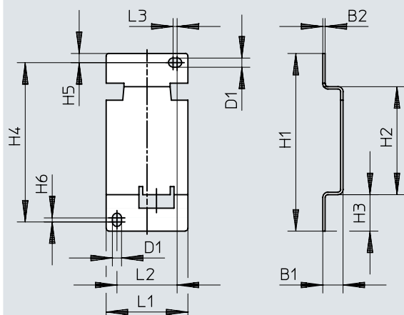
Dimensões – Placa adaptável SDE1- ...-W ...
