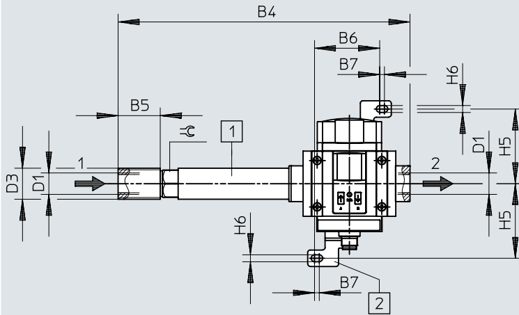
치수 - 단일 장착용 SFAM-62-...-T/W
