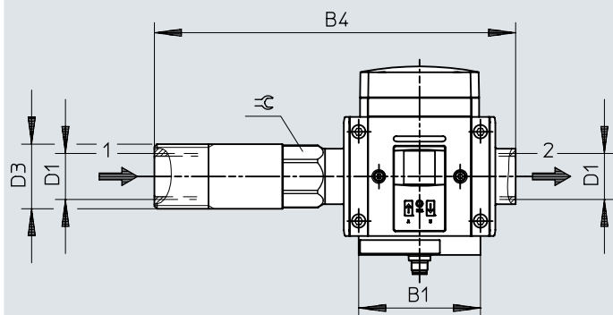
치수 - 단일 장착용 SFAM-90-...-T
