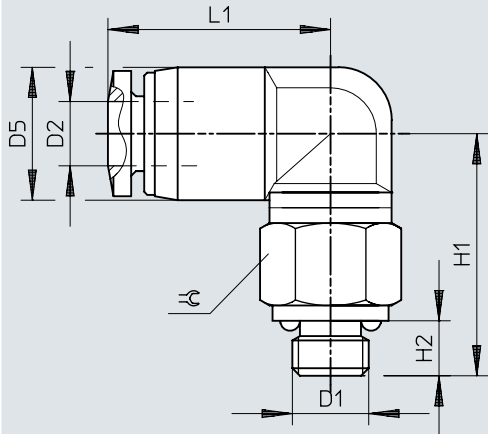
치수 - L 푸시인 피팅 QBML, UNF 나사산
