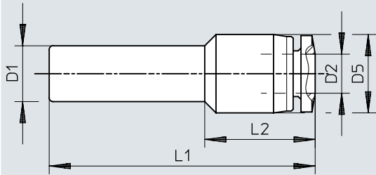
치수 - 플러그 커넥터 QBM-...H
