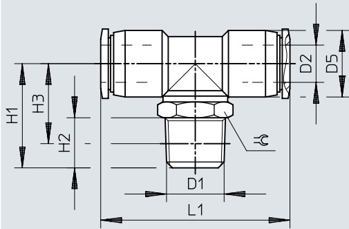
치수 - T 푸시인 피팅 QBMT, NPT 나사산
