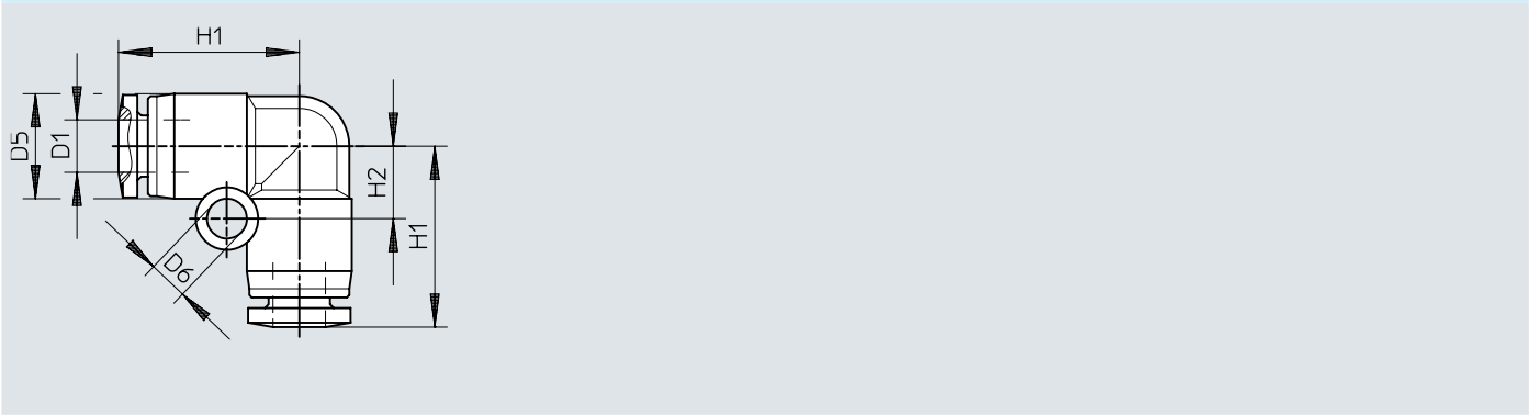
치수 – 푸시인 L-커넥터 QBML-...T
