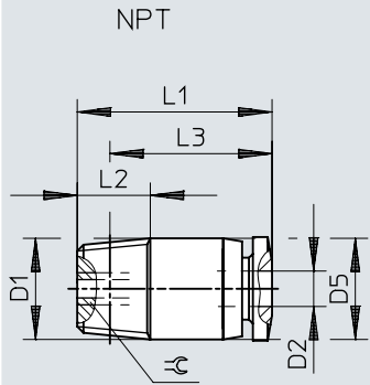
치수 – 푸시인 피팅 QBM-...-I, NPT 나사산
