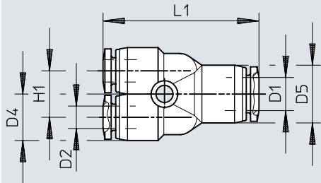
치수 – 푸시인 Y-커넥터 QBM...T, 감소
