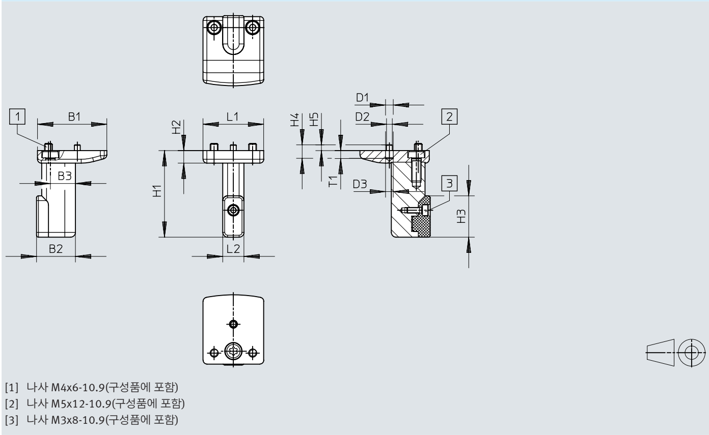
치수 - 그리퍼 핑거 HAFH-B30-16-45-N
