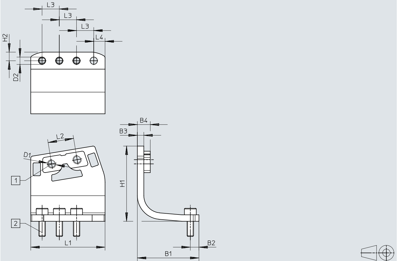
치수 - 마운팅 브라켓 DHAS-MA-B6-80
