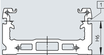
外形寸法図 - ELGD-TB-_- (フレーム)
