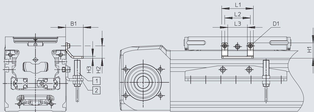
外形寸法図 - センサドグ EAPM-E24-_-SLE
