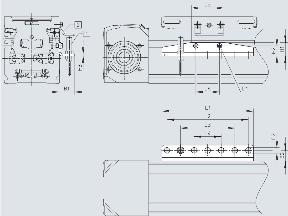
外形寸法図 - センサブラケット EAPM-E24-60-SHE
