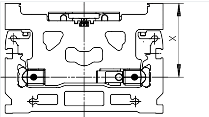
テーブル面からガイド中心までの距離
