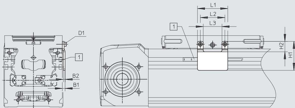
外形寸法図 - センサドグ EAPM-E24-60-SLS
