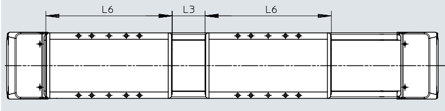
外形寸法図 - ELGD-TB-_-ZL/-ZR(追加テーブル)
