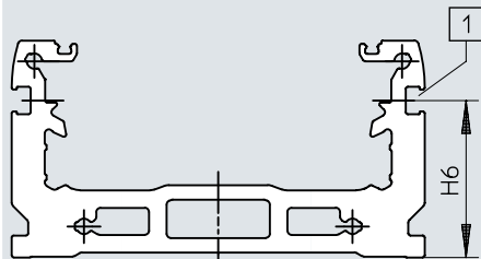
外形寸法図 - ELGD-TB-_- (フレーム)
