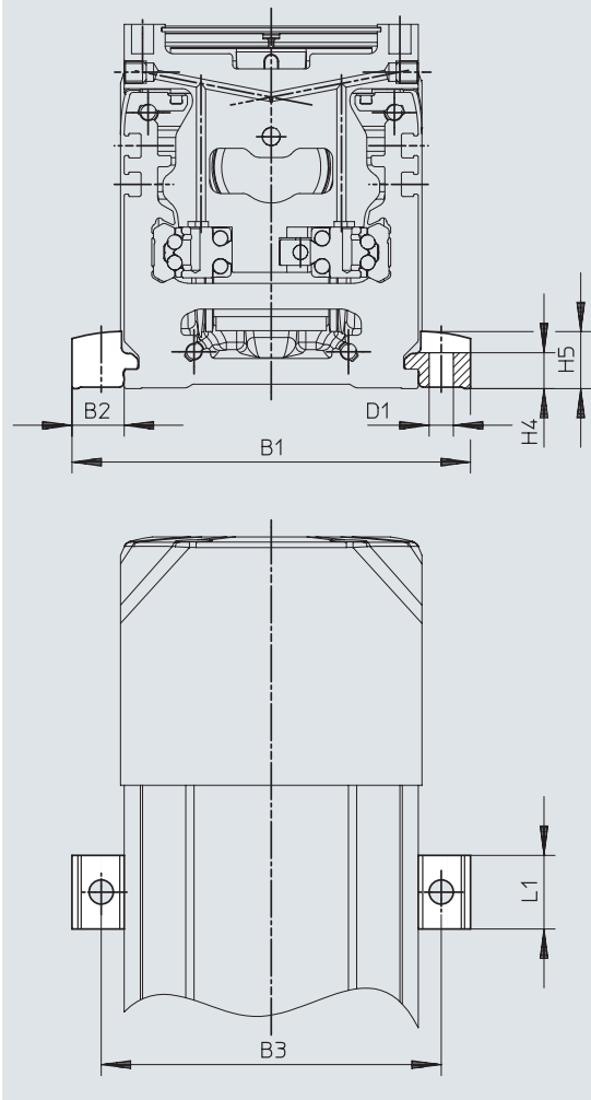
外形寸法図 – 本体取付金具 EAHF-E24-60-P-S
